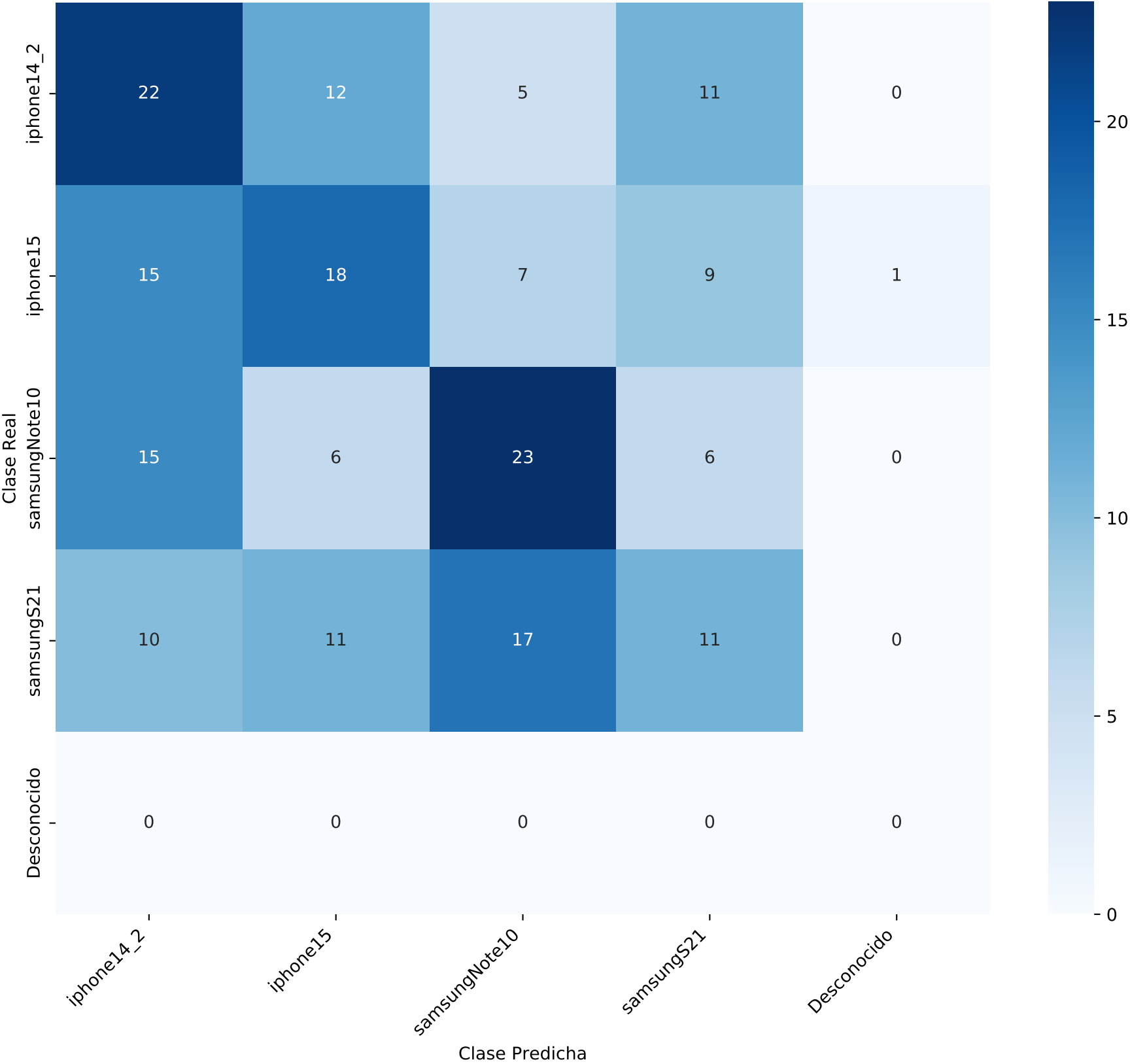
Matriz de Confusión - PRNU_BLANCO Y NEGRO
